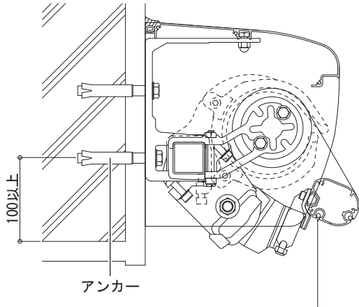
[1] コンクリート造壁面納まり
