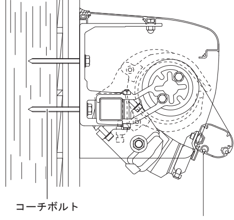
[2] 木造壁面納まり
