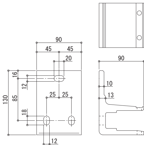
[1] 壁付用取付ブラケット
