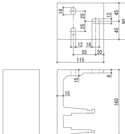
[4] 上ケース用補助取付ブラケット
