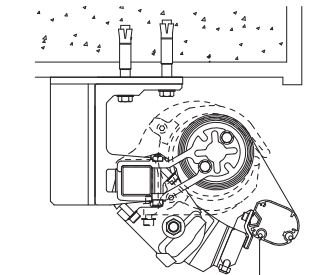
b タイプ補助金具納まり図
