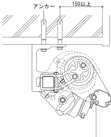
[4] コンクリート造天井納まり
