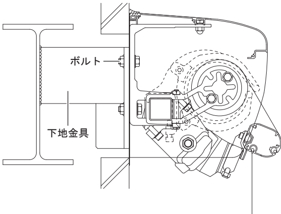
[3] ALC 造壁面納まり
