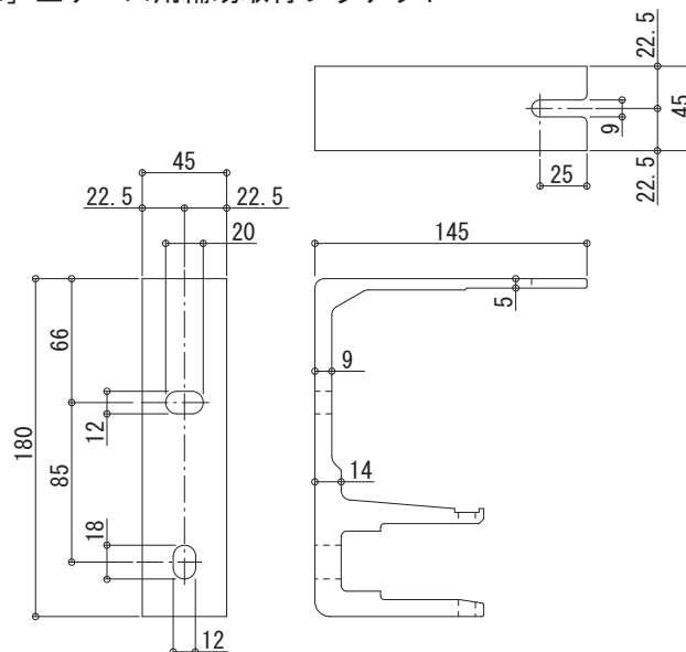
[4] 上ケース用補助取付ブラケット
