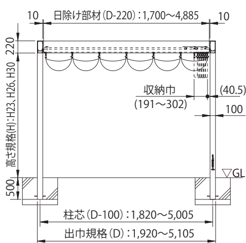
【単装サイズ】
