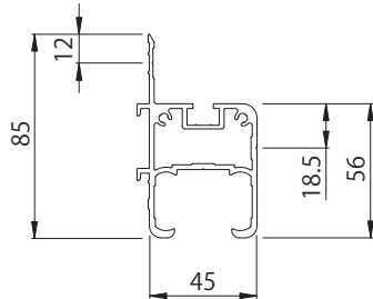
【レール断面】
