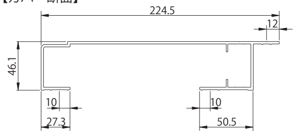
【カバー断面】
