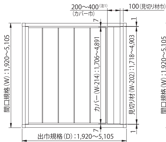
【単装サイズ】
