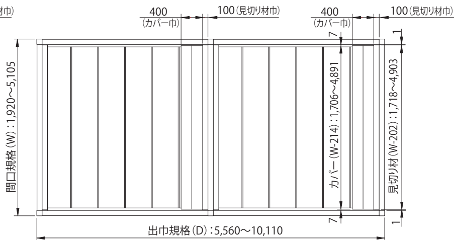
【連棟サイズ】
