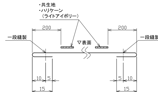
B-B断面図
