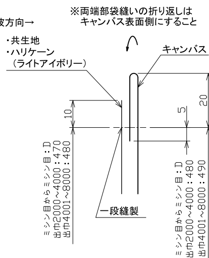
袋部断面図
